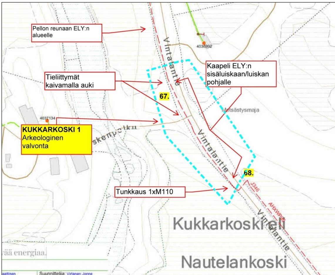
Tilajan maastosuunnitelmapartta. Muinisjäännösalueen pohjoisin osa on valvottavaksi määritellyn osan ulkopuolella.
