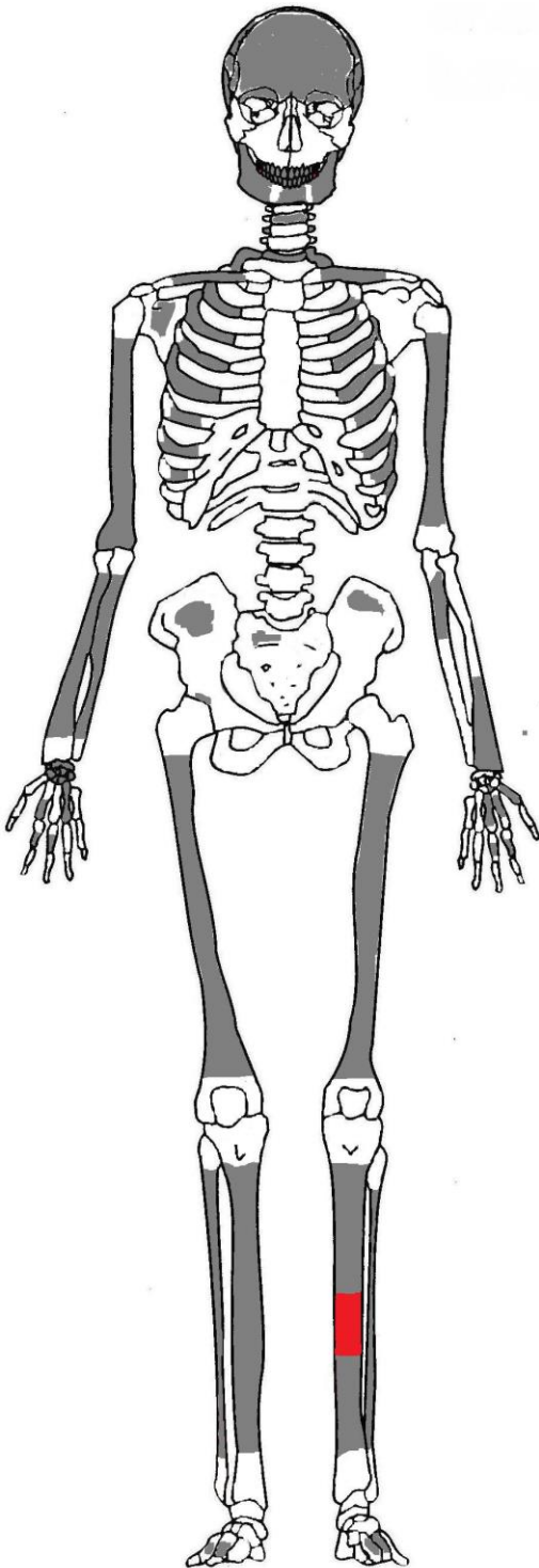
Kuva 13. Uudelleen luutunut sääriluu
