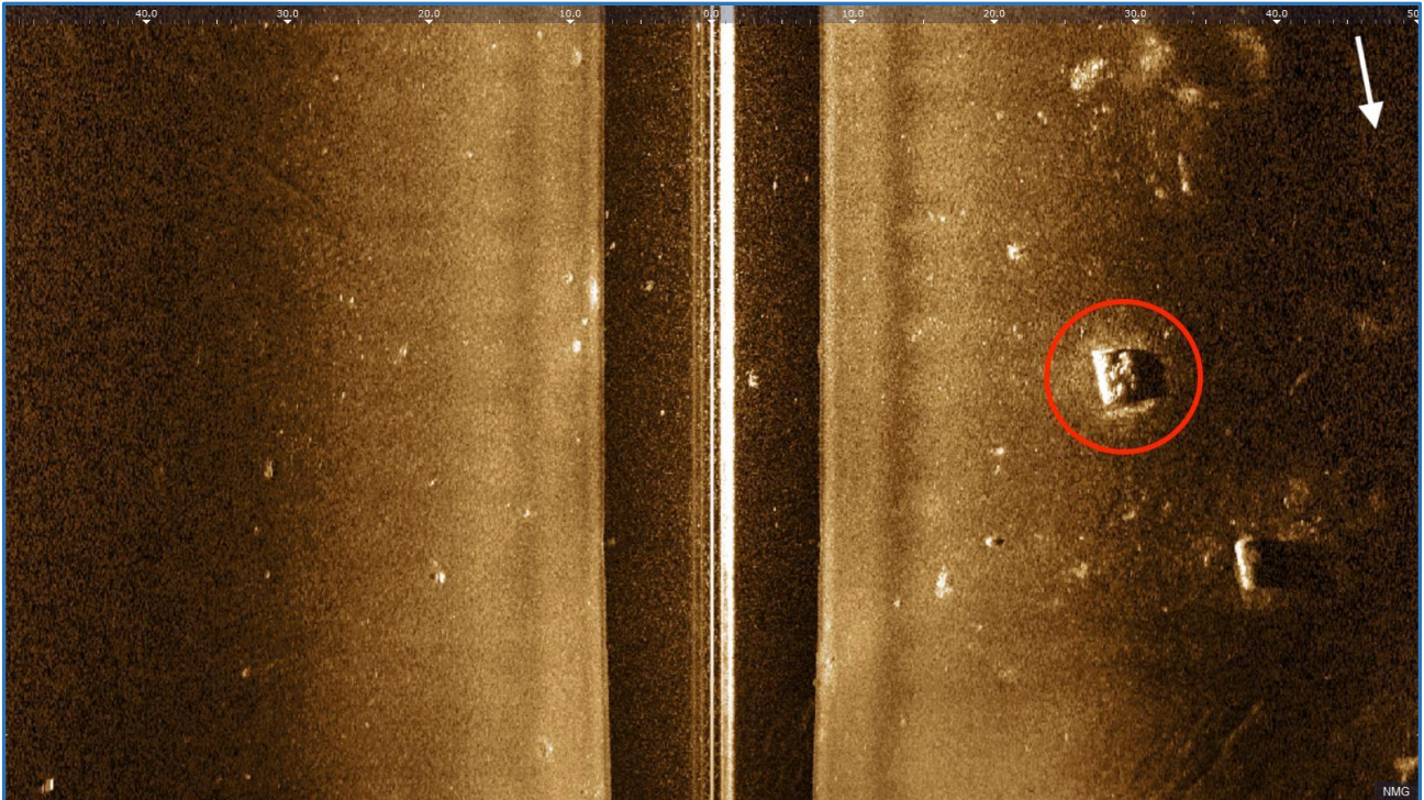
Kuva 4. Viistokaikuluotauskuva kohteesta 2. Mahdollinen hirsiarckku.
