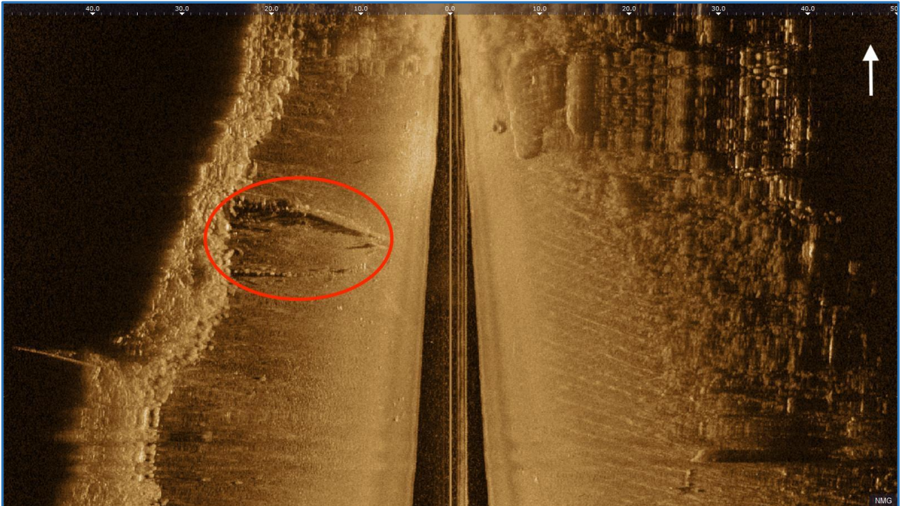
Kuva 5. Viistokaikuluotauskuva kohteesta 3. Todennäköisesti kyseessä on kaksi putkilinjaa, mutta niitä ei ole merkitty moderneihin karttoihin.
