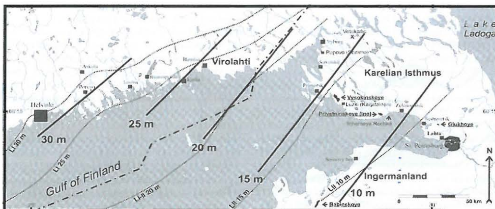
Kuva 3. Litorinameren transgression korkeimman rantatason isobaasit Miettisen mukaan. Hyyppän (1937) esittämät isobaasit on merkitty pisteiviivoilla (Miettinen 2002: Fig.50).
