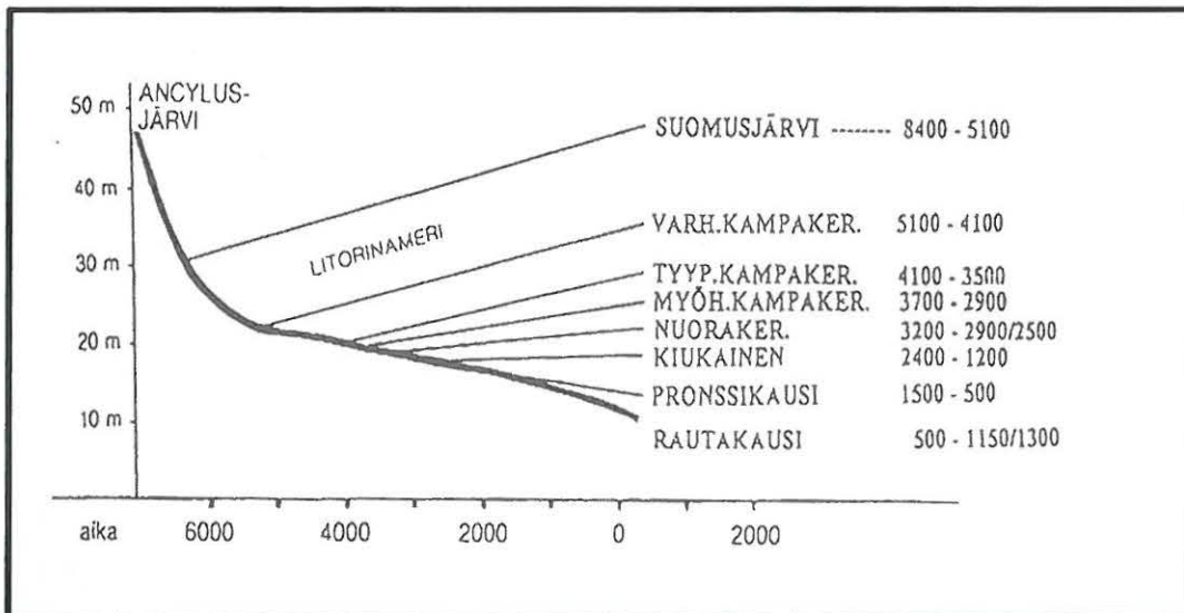
Kuva 4. Yksinkertaistettu rannansiirtymiskäyrä muinaisjännösten kytkeytymisestä muinaisiin rantapintoihin Kymenlaakson rannikolla (Miettinen 1998:12).
