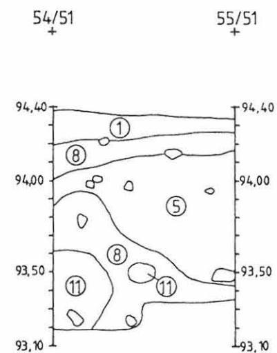
Länsileikkaus
