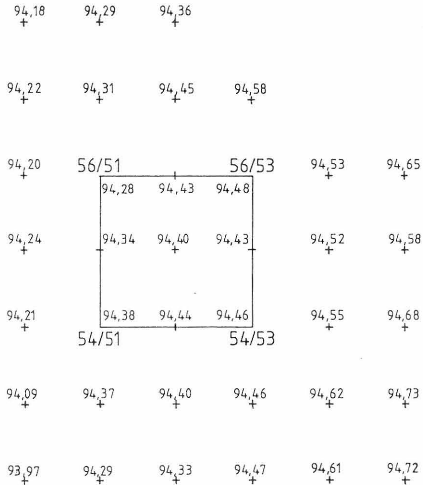
pintavaaitus
