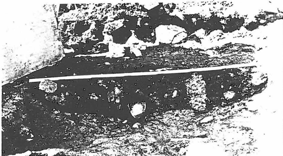
Ruudun 562/402 tulisijan etelä-pohjoissuuntainen leikkaus, kuvattu idästä.
