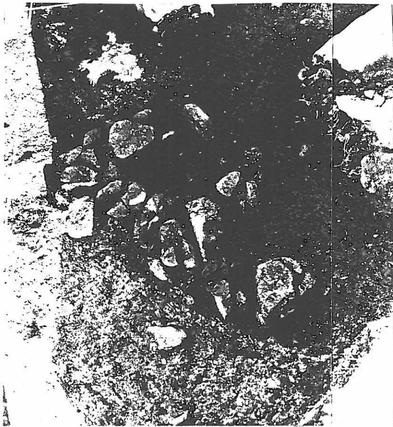
Tulisijan kiveystä ruudussa 562/406, kuvattu idästä.
