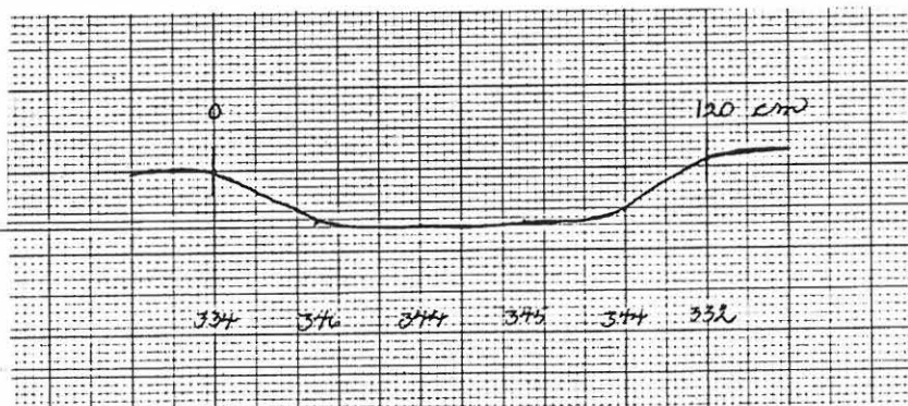
Ruudun 562/402 tulisijan etelä-pohjoissuuntainen leikkaus, kuvattu idästä.
