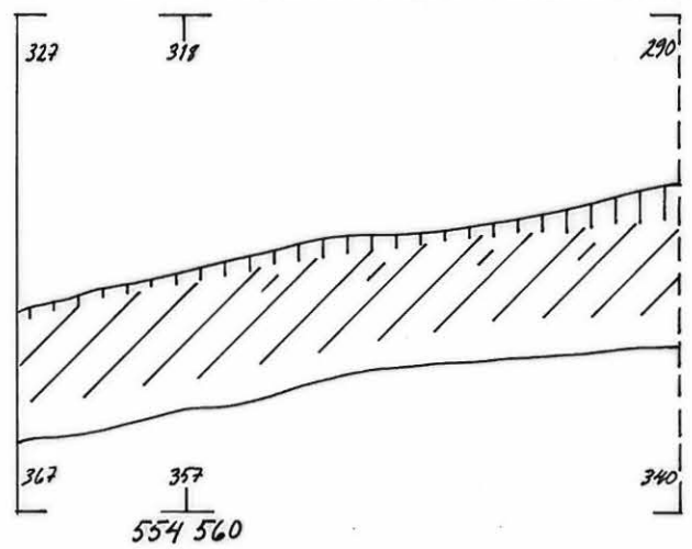
ITA'-LANSI SUUNTAINEN PROFIILI LINJALLA 554 POHJOISESTA
