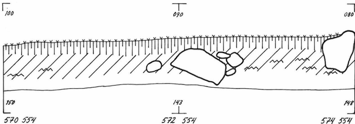
POHJOIS-ETELÄ SUUNTAINEN PROFIILI LINJALLA 554 IDÄSTÄ
