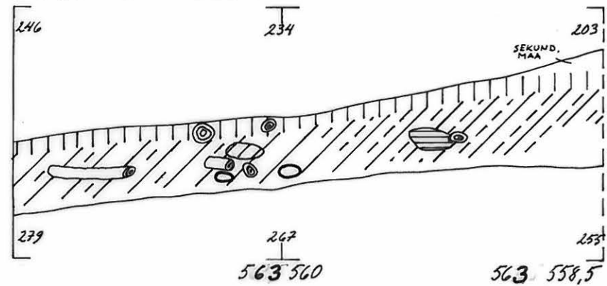
ITÄ-LÄNSI SUUNTAINEN PROFIIILI LINJALLA 562,5 POHJOISESTA
