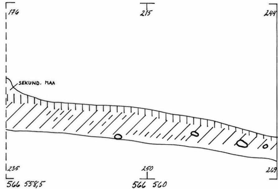
ITÄ-LÄNSI SUUNTAINEN PROFIIILI LINJALLA 566 ETELÄSTÄ
