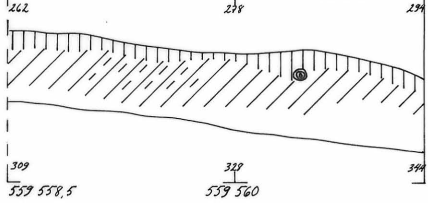
ITA'-LANSI SUUNTAINEN PROFIILI LINJALLA 559 ETELASTA
