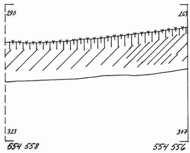
ITA'-LANSI SUUNTAINEN PROFIILI LINJALLA 559 ETELASTA
