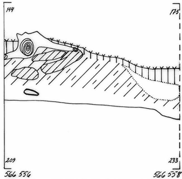
ITÄ-LÄNSI SUUNTAINEN PROFIIILI LINJALLA 566 ETELÄSTÄ
