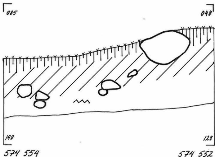
ITÄ-LÄNSI SUUNTAINEN PROFIILI LINJALLA 574 POHJOISESTA
