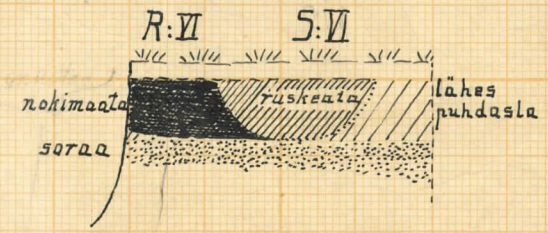
Tulisija \delta , poikkileikkaus 9-10 2 cm = 1 m.
