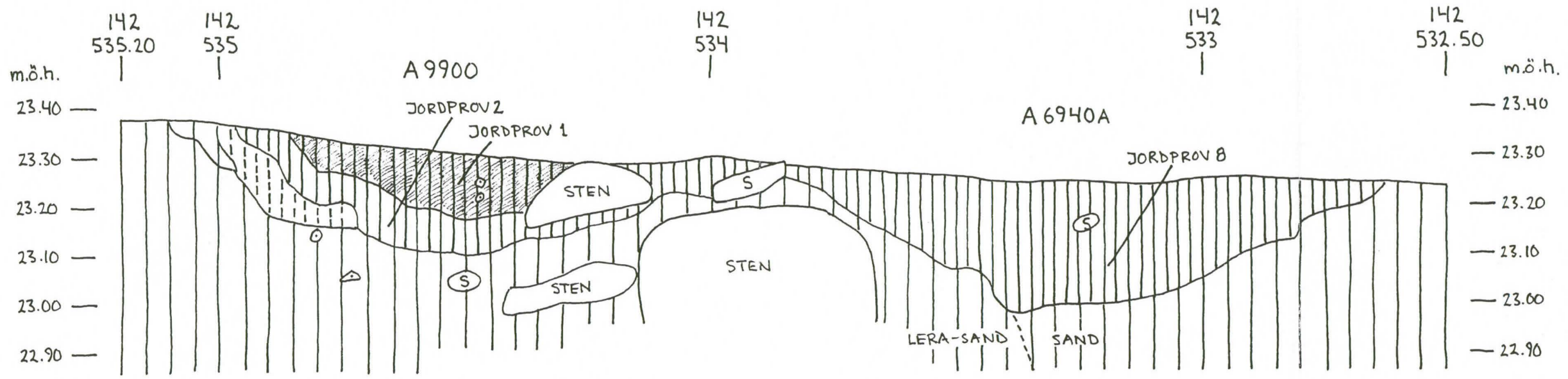
VÖRÅ, PÖRNULLBACKEN, ANL. 6940A PROFIL 8 & ANL. 9900 FRÅN N, SKALA 1:10, MARINA ANDERSSON, 99.07.19
