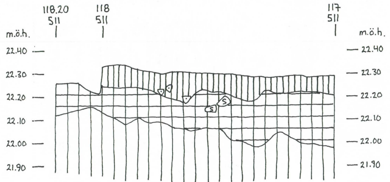
VÖRÅ, PÖRNULLBACKEN, ANL. 9040 & 9060 PROFIL 2 FRÅN V, SKALA 1:10 99.07.09 LINDA GRANFORS & JONAS FORTH
