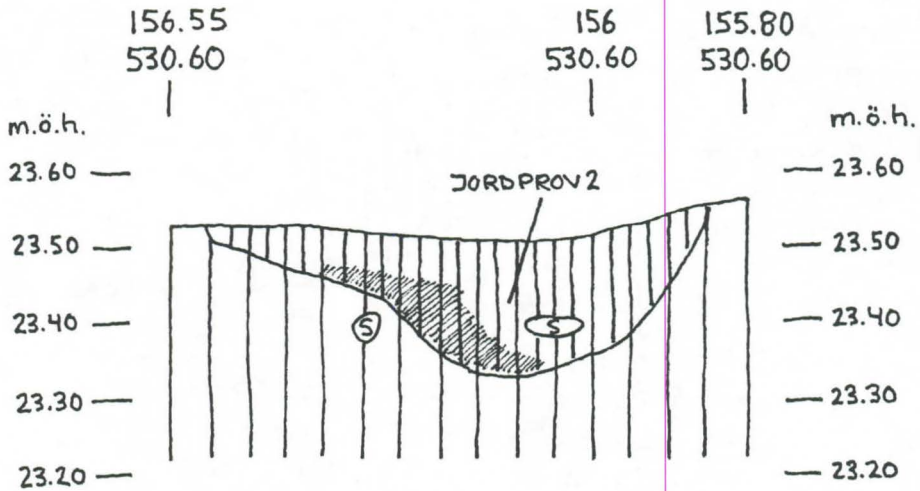
VÖRÅ, PÖRNÜLLBACKEN, ANL. 10800 PROFIL 1 FRÅN V, SKALA 1:10 MARINA ANDERSSON, 99-08-02
