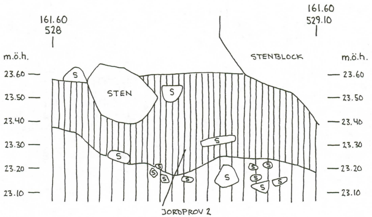
VÖRÅ, PÖRNULBACKEN, ANL. 10860 A, PROFIL 2 FRÅN S SKALA 1:10, CHARLOTTA HELGESSON, 99.08.04
