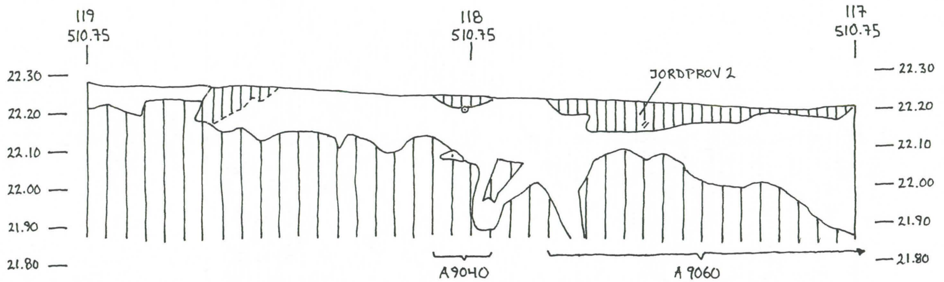
VÖRÅ, PÖRNULLBACKEN, ANL. 9040 & 9060, PROFIL 1 FRÅN V, SKALA 1:10 99.07.08 LINDA GRANFORS & JONAS FORTH
