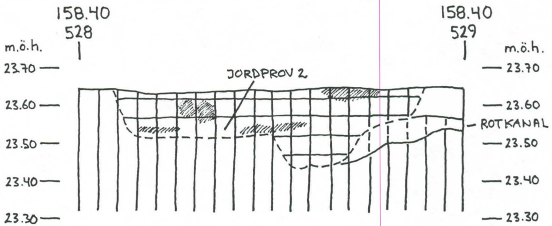
VÖRÅ, PÖRNÜLLBACKEN, ANL. 10920, PROFIL 1 FRÅN S, SKALA 1:10, JONAS FORTH, 99.07.27
