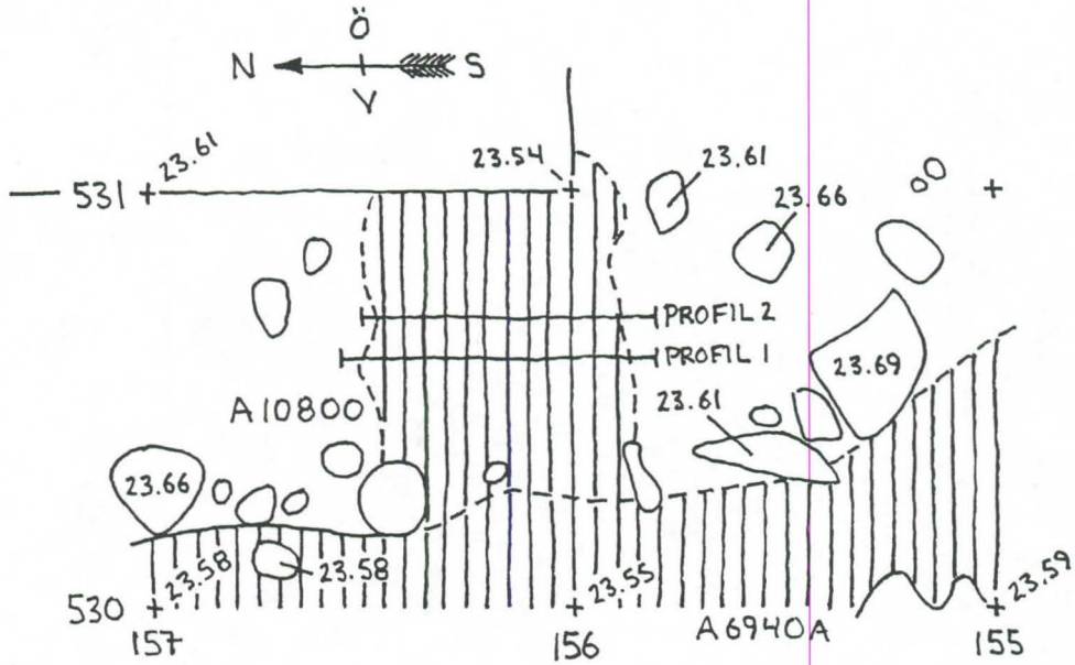
VÖRÅ, PÖRNÜLLBACKEN, ANL. 10800, SKALA 1:20
