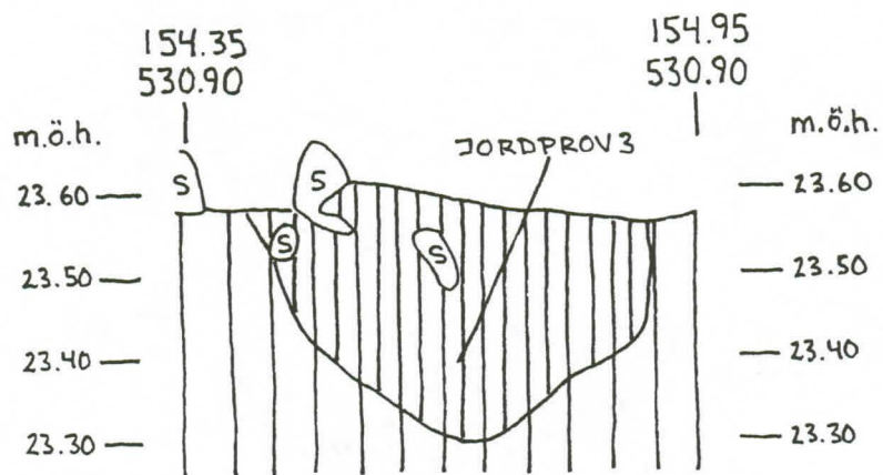
VÖRÅ, PÖRNULLBACKEN, ANL. 10780 PROFIL 2 FRÅN Ö, SKALA 1:10 MARINA ANDERSSON, 99.07.26
