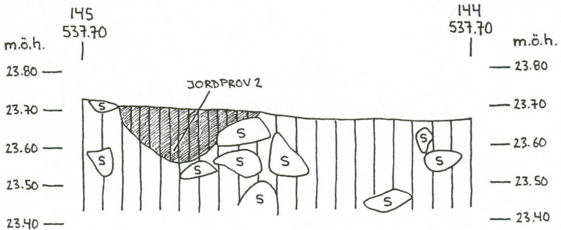
VÖRÅ PÖRNÜLLBACKEN ANL. 9760 PROFIL FRÅN V SKALA 1:10 MAHMOOD SAL 99.07.06
