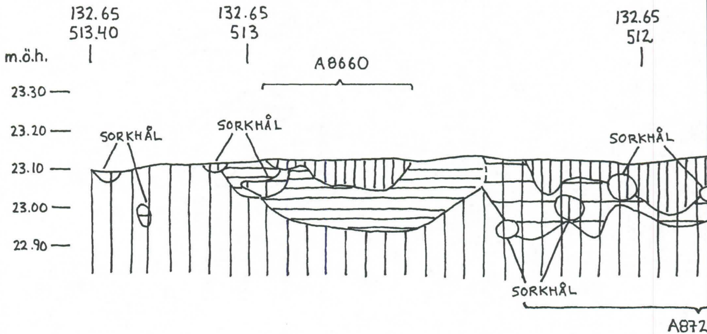
VÖRÅ, PÖRNULLBACKEN, ANL. 8660 & 8720, PROFIL 3 FRÅN
