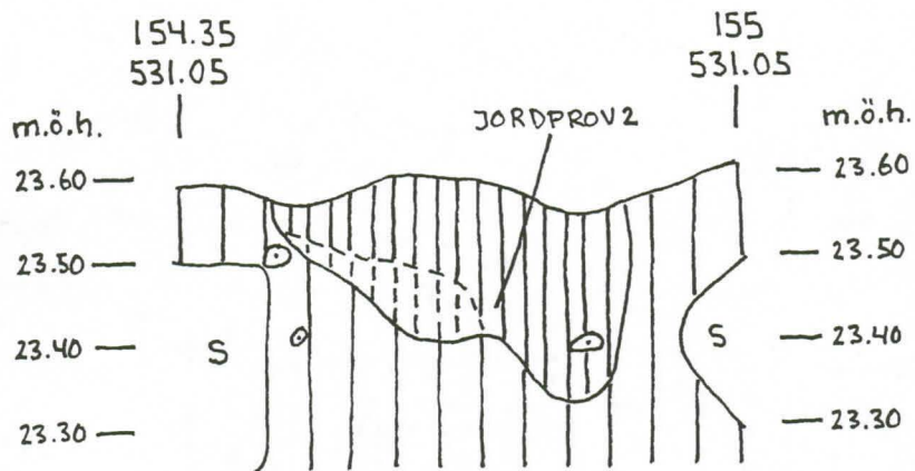
VÖRÅ, PÖRNULLBACKEN, ANL. 10780 PROFIL 1 FRÅN Ö, SKALA 1:10 MARINA ANDERSSON, 99.07.26
