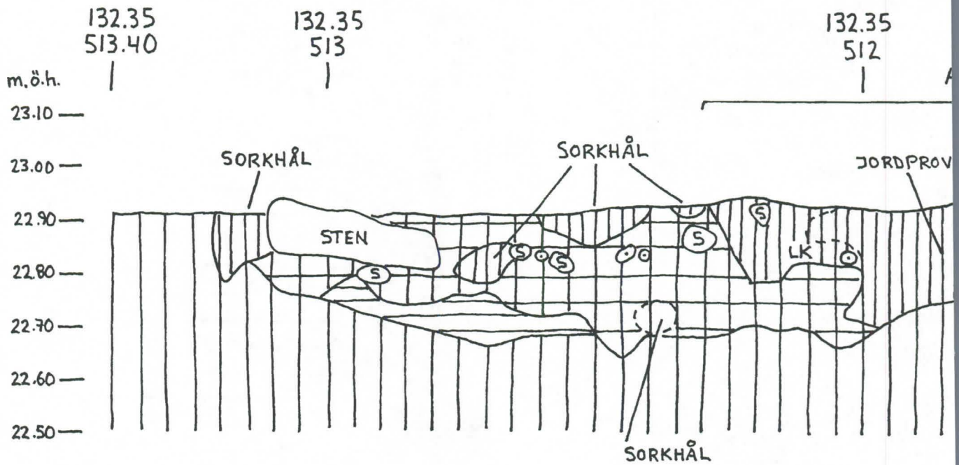
VÖRÅ, PÖRNULLBACKEN, ANL. 8680 & 8720, PROFIL 4 FRÅN
