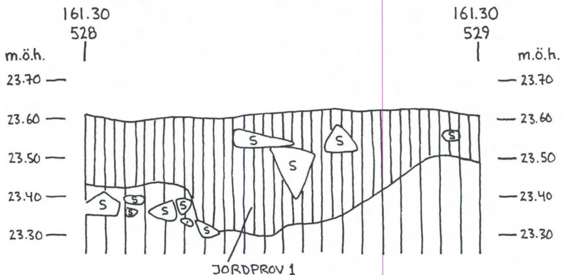
VÖRÅ PÖRNULLBACKEN ANL. 10860A PROFIL 1 FRÅN S SKALA 1:10 CHARLOTTA HELGESSON 99.08.04
