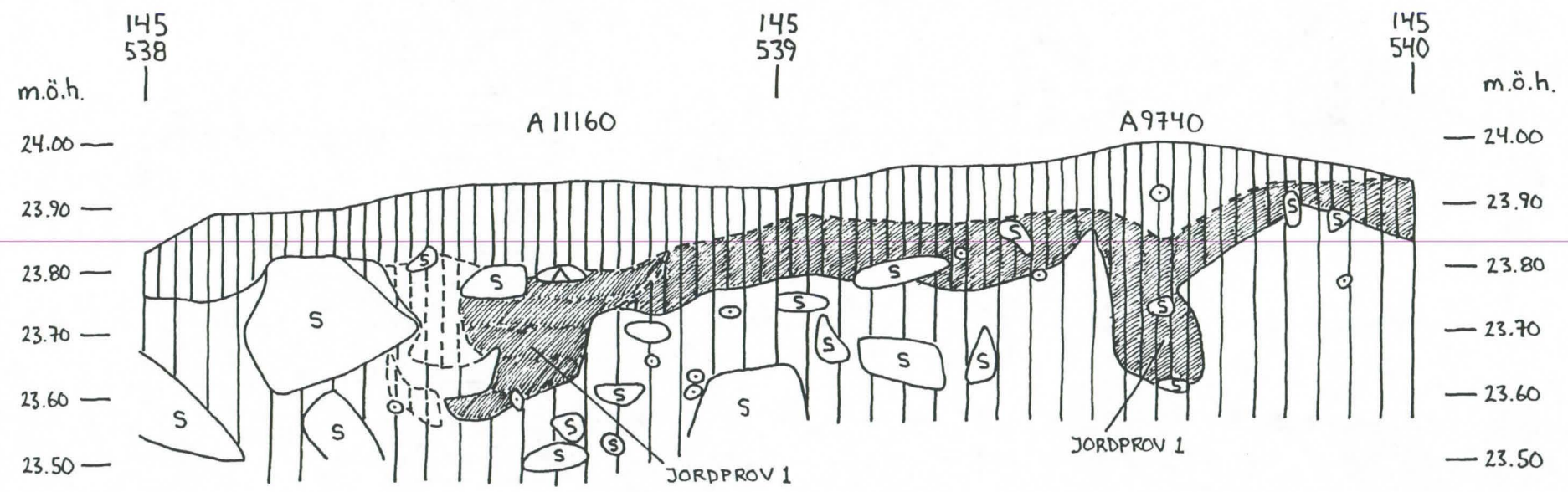
VÖRÅ, PÖRNULLBACKEN, ANL. 9740 & 11160, PROFIL FRÅN S, SKALA 1:10, MIRJAM JONSSON, 99.08.04
