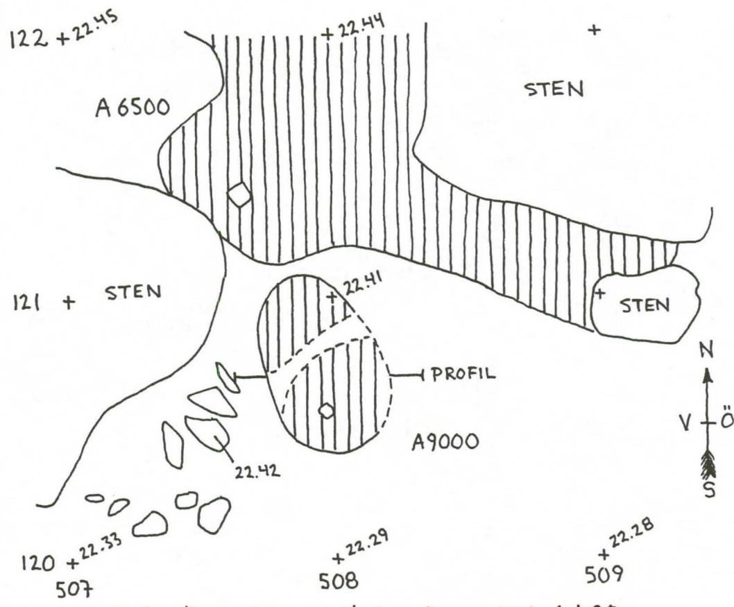
VÖRÅ, PÖRNÜLLBACKEN, ANL. 9000, SKALA 1:20
