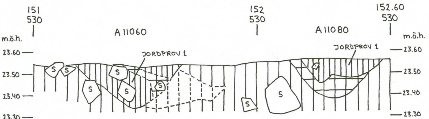
VÖRÅ PÖRNULLBACKEN ANL. 11060 & 11080 PROFIL FRÅN Ö SKALA 1:10 JONAS FORTH 99.07.28
