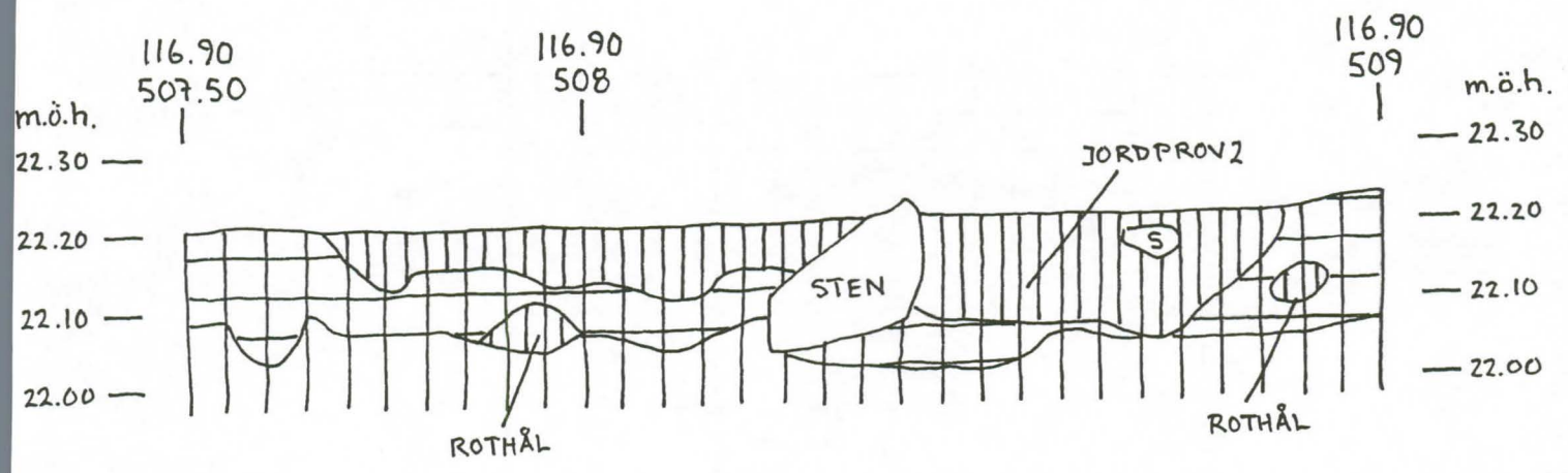
VÖRÅ PÖRNULLBACKEN ANL. 9100 PROFIL FRÅN S SKALA 1:10 99.07.14 MAHMOOD SAL
