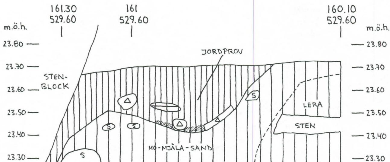
VÖRÅ, PÖRNULLBACKEN ANL. 10860 B PROFIL 1 FRÅN V SKALA 1:10 CHARLOTTA HELGESSON 99.08.03
