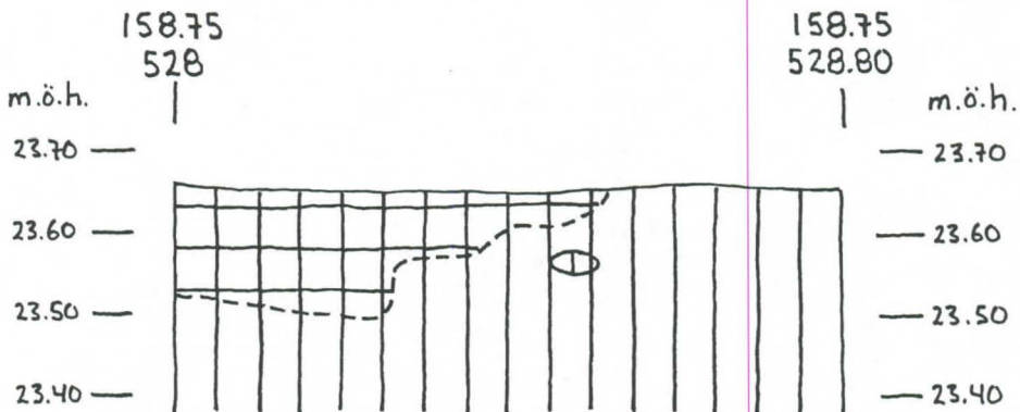
VÖRÅ, PÖRNÜLLBACKEN, ANL. 10920 PROFIL 2 FRÅN S, SKALA 1:10 JONAS FORTH, 99.07.27
