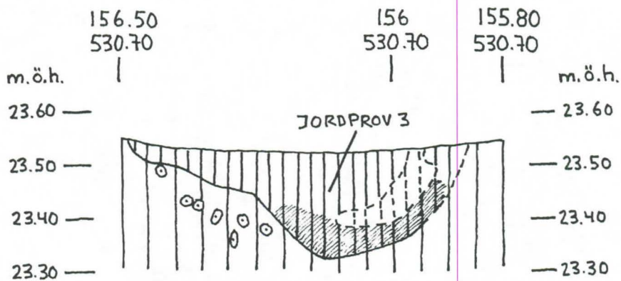
VÖRÅ, PÖRNÜLLBACKEN, ANL. 10800 PROFIL 2 FRÅN V, SKALA 1:10 MARINA ANDERSSON, 99-08-02
