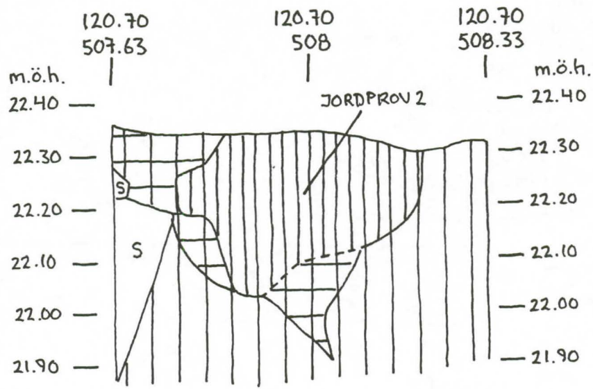
VÖRÅ PÖRNÜLLBACKEN ANL. 9000 PROFIL FRÅN 5 SKALA 1:10 99.07.14 LINDA GRANFORS & JONAS FORTH
