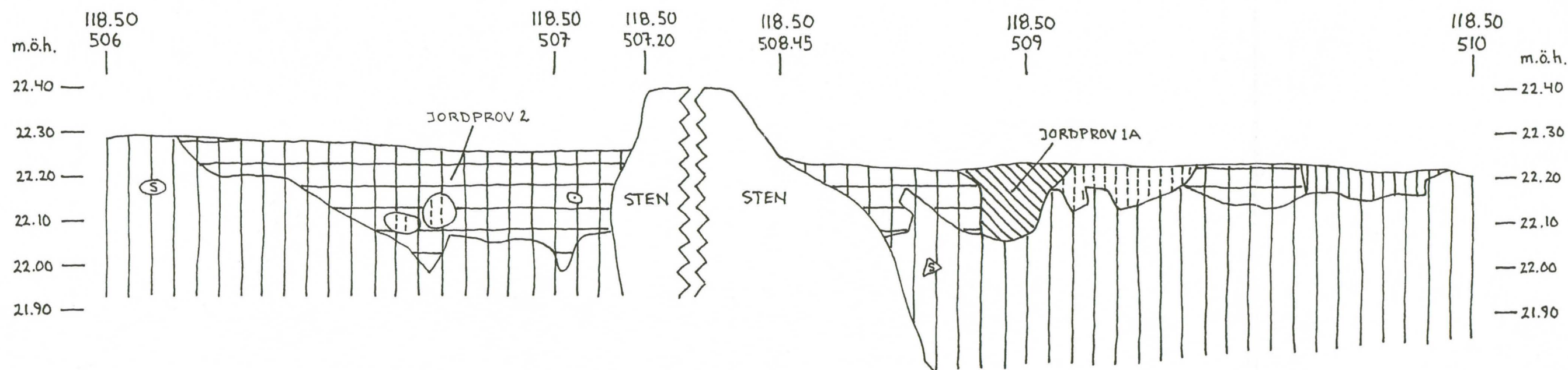
VÖRÅ, PÖRNULLBACKEN, ANL. 6520, PROFIL 1 FRÅN S, SKALA 1:10, 99-07-12, LINDA GRANFORS, JONAS FORTH & LAURI SKANTSI
