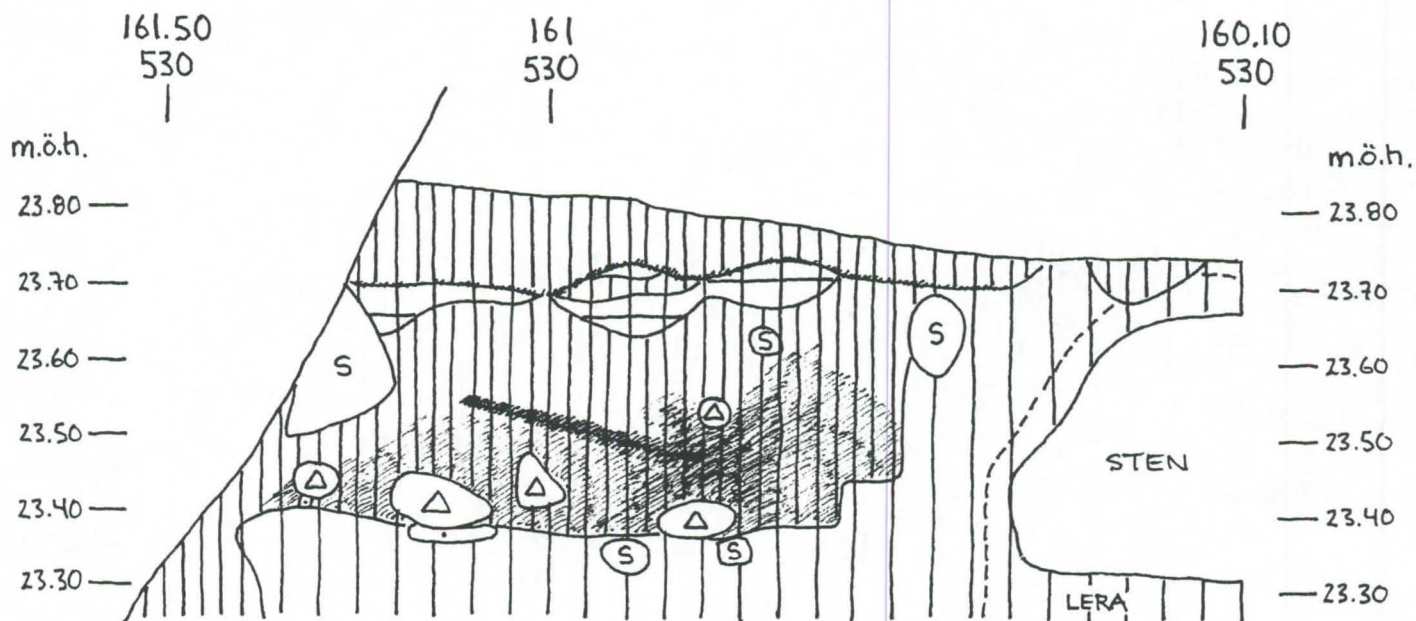
VÖRÅ, PÖRNULLBACKEN ANL. 10860 B PROFIL 2 FRÅN V SKALA 1:10 CHARLOTTA HELGESSON 99.08.03
