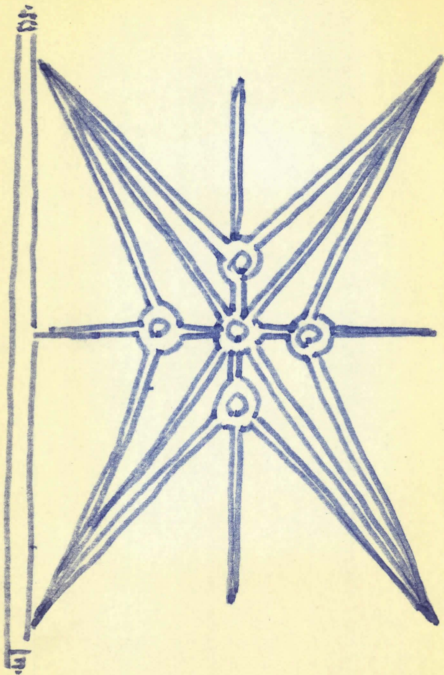
Fig. 9 Västra valvet
