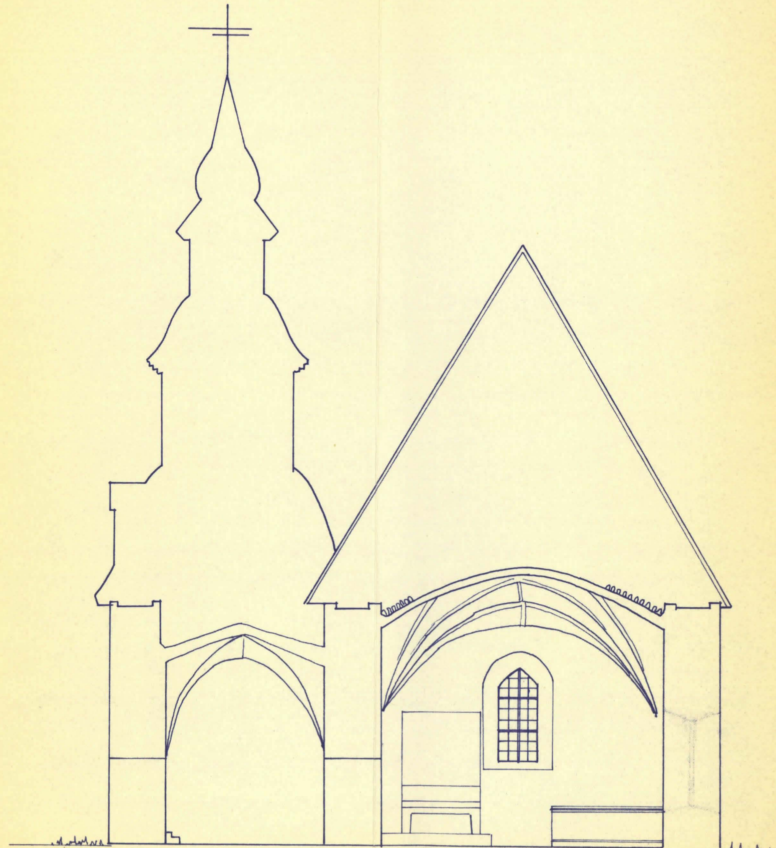
SKÄRNING B - B
