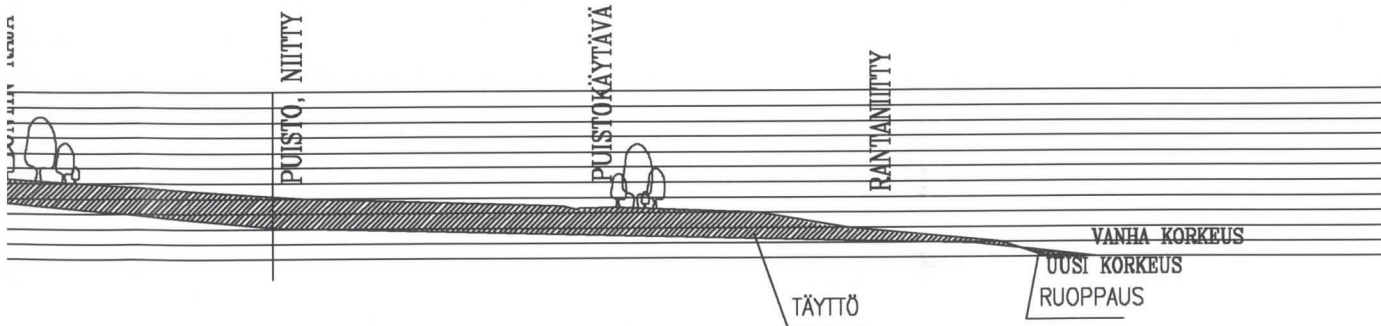
POIKKILEIKKAUS B
