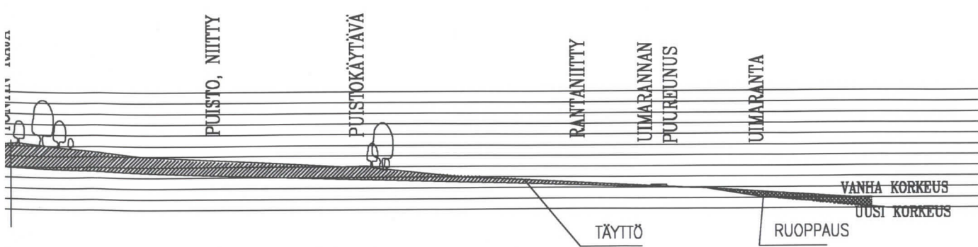
POIKKILEIKKAUS A
