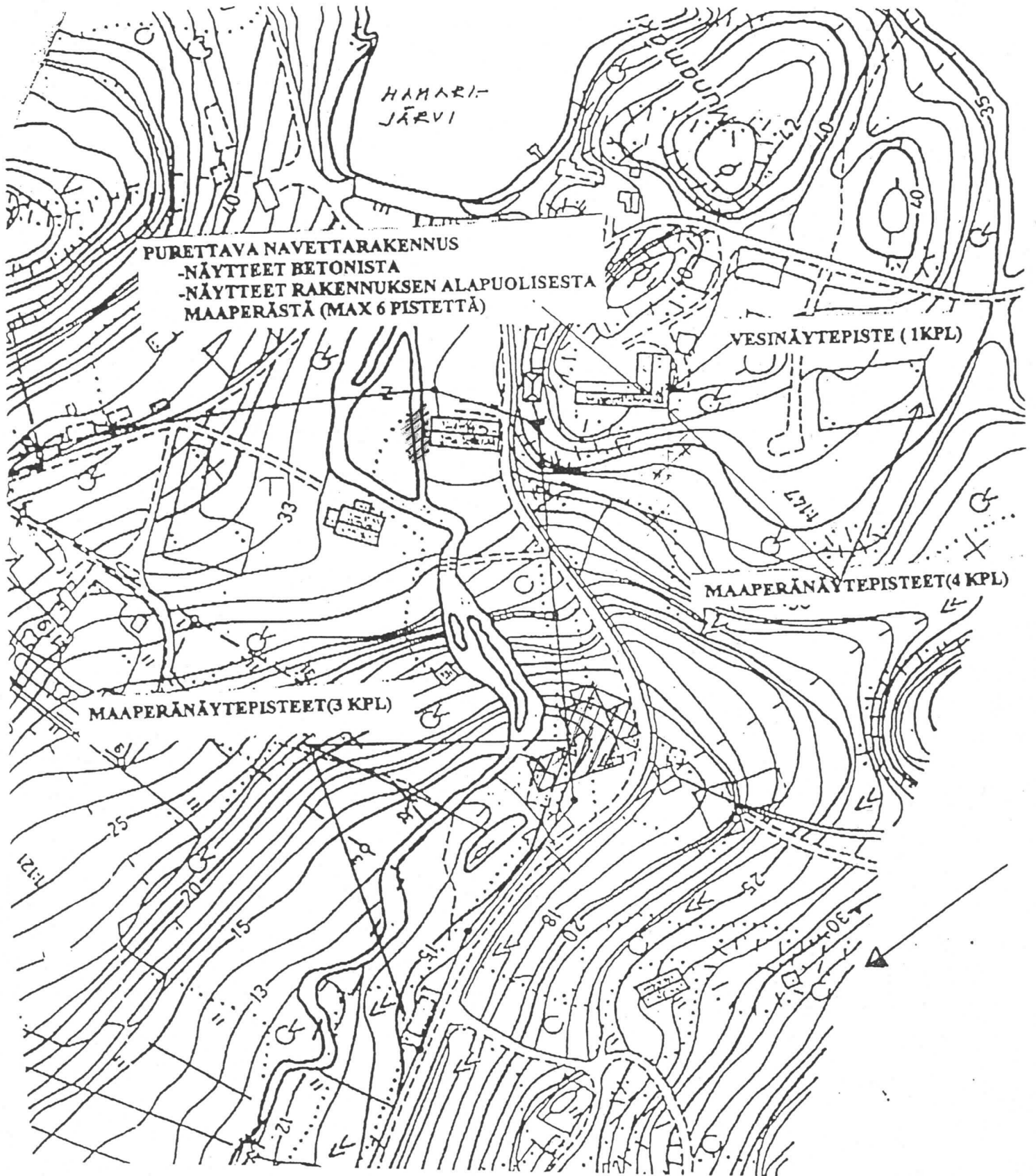
PERNIÖ KIRJAKKALA Vedenjohtokanaalin perkaus Karttaote 1:2000
