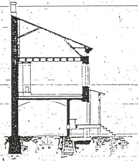
Gemenskärning i A.B.
