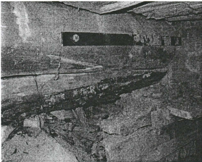
Kuva 1. Betonipalkkiin pultattu vanhaa lattiaa kannatteleva niskahirsi kammion 14 länsipuolella (125612: 117).
