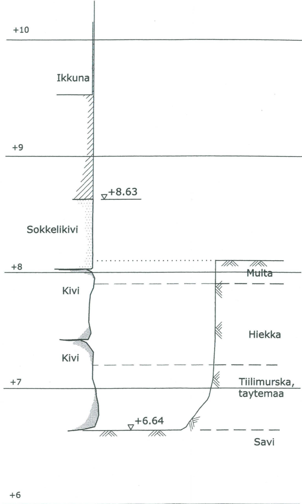
Koekuoppa 2 Leikkaus B - B, 1:20
