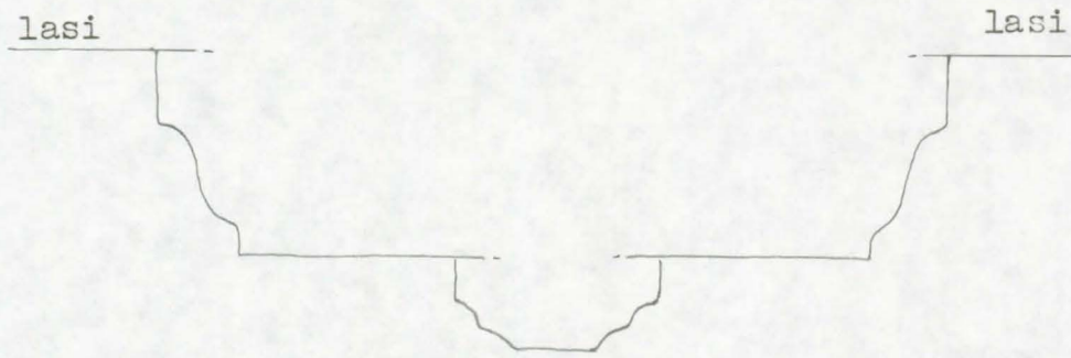
Ikkunapuitteiden keskiosa
