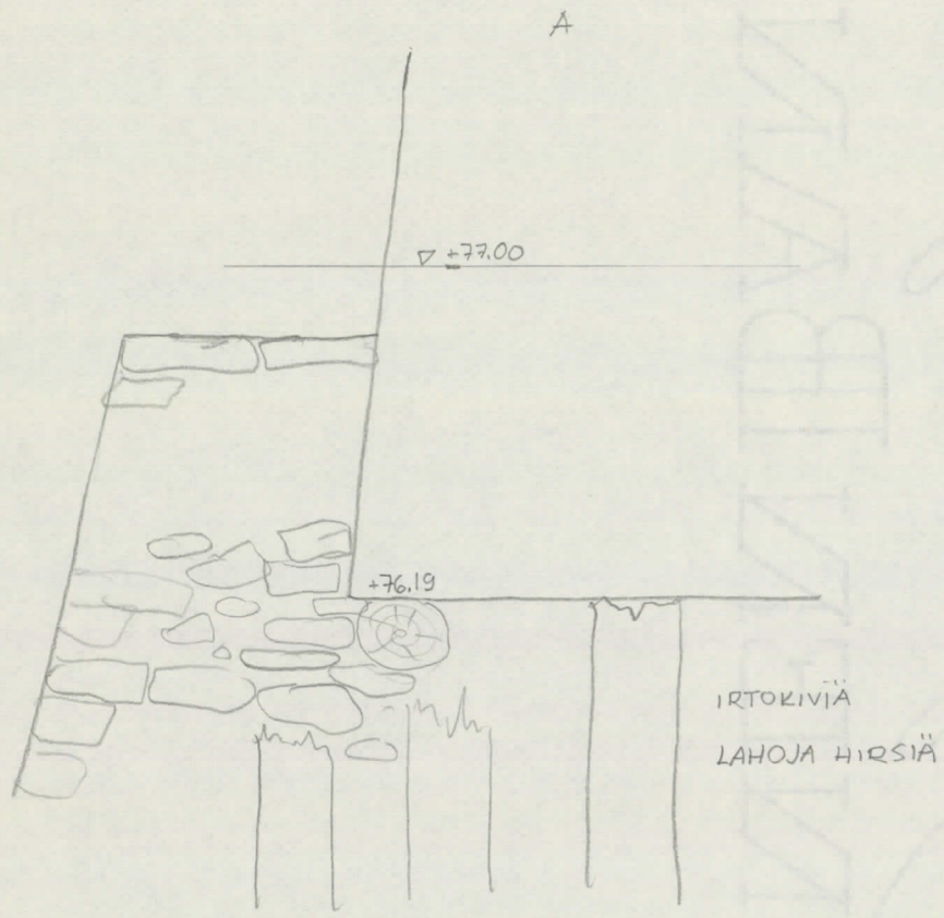
SUVOROV, PITKÄ ITÄSIIVY KAAVAKUVA MK. N. 1:20
