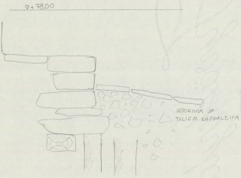
PÄÄPORTIN LAITURIN VASEMMAN OSAN (LUOTEISSIVU) POIKKILEIKKAUS, KAAVAKUVA MK. 1:20
