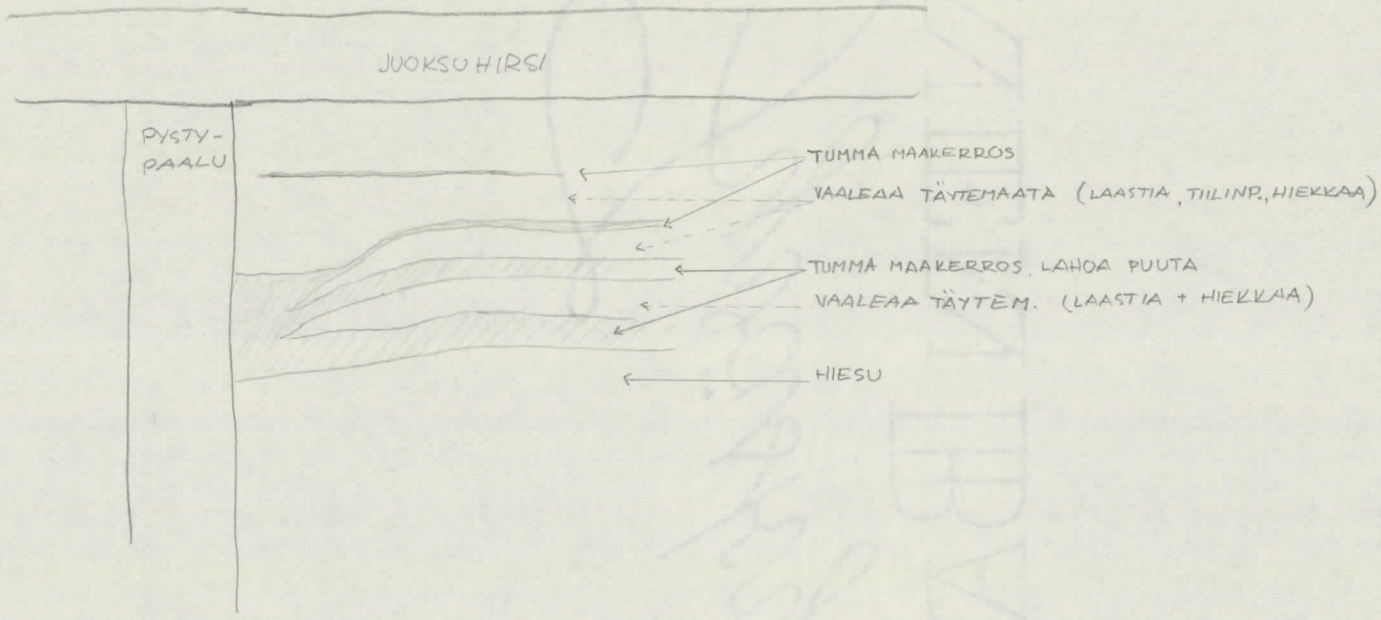
PÄÄPORTIN OIKEAN PIELEN (KAARKKOISP.) ANTURAN KAIVANTO KAAVAMAINEN ESITYS MAAKERROKSISTA MUURIN ALLA. MK. 1:20
