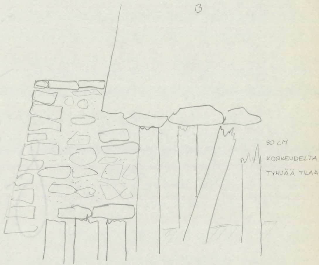
SUVOROV, LYHYT ITÄSIIVY, POHJOISPÄÄ, KAAVAKUVA MK. N. 1:20
