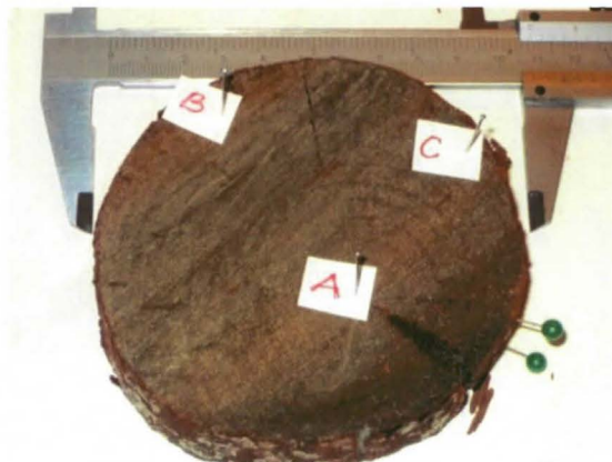
Kuva 5.23. Raakapuunäytteestä sahattu kiekko ilmakeivatuksen jälkeen. Mitatut kutistumissuunnat puun poikkileikkaussuunnassa: A-B (ja A-C) = radiaalinen, B-C = tangenciaalinen. Vihreät neulat = pituussuuntainen. Kuva Rami Kokko, Museovirasto.
