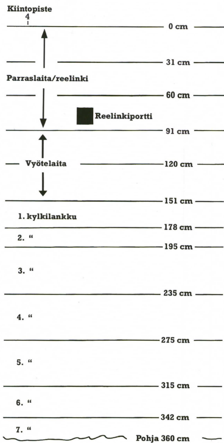
Kuva 5.2.4. Mittatiedot hylyn paapuurinpuoleisen parraslaidan/reelingin ylätasosta pohjaan kiintopiste 4:n kohdalta mitattuna. Piirros Rami Kokko, Museovirasto.
