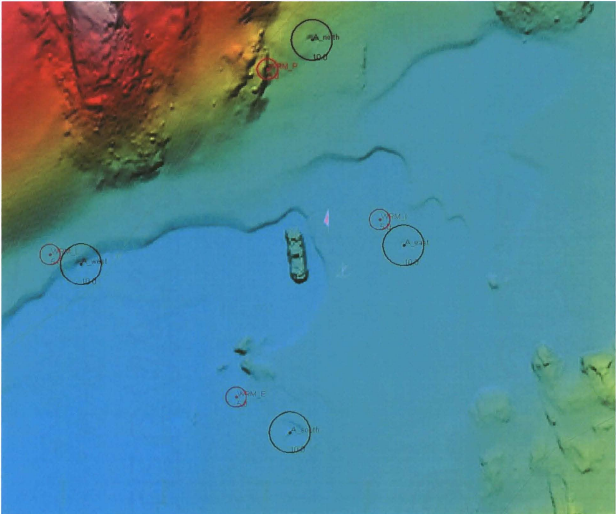
Kuva 3.2. Alkuperäisten poijupainojen sijainnit Vrouw Maria-hylyn ympärillä (mustat ympyrät). Uudet painot on laskettu alkuperäisten painojen välittömään läheisyyteen uutta itä-painoa lukuun ottamatta. Itä-paino on siirretty n. 50 m itään päin kuvan osoittamasta idänpuoleisesta ympyrästä. Kuva Meritaito Oy (MA201014:65).
