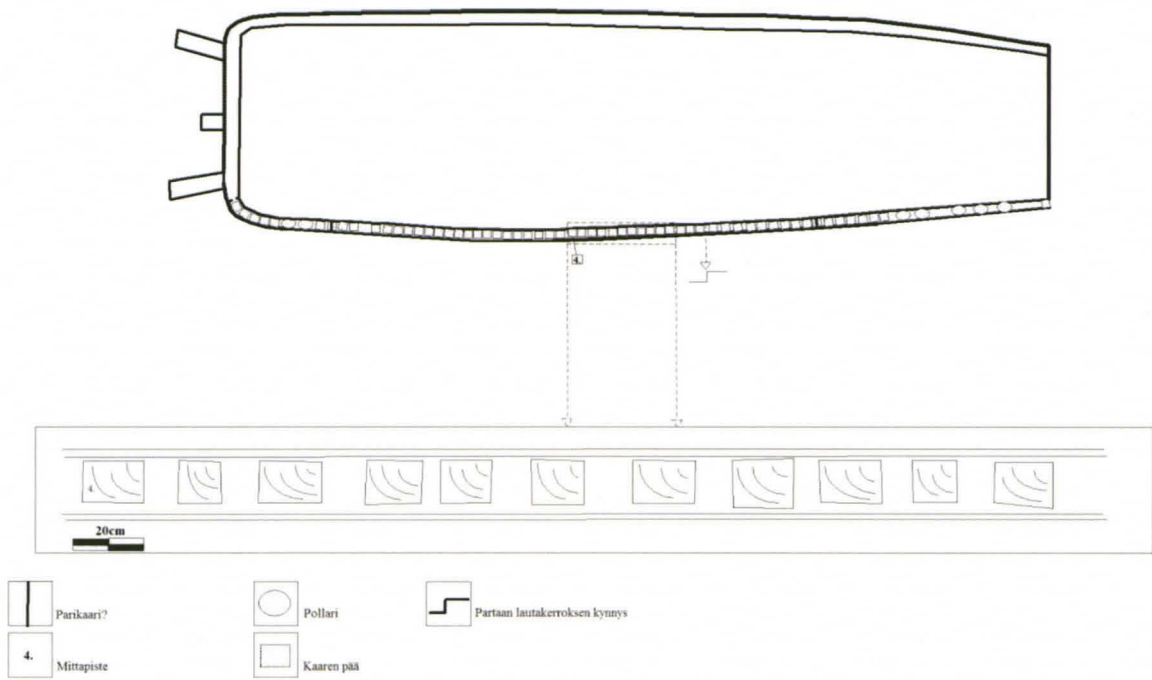
Kuva 5.2.2. Mitatut kaarivälit paapuurin puoleisella parraslaidalla. Kuva RiikkaTevali, Museovirasto.
