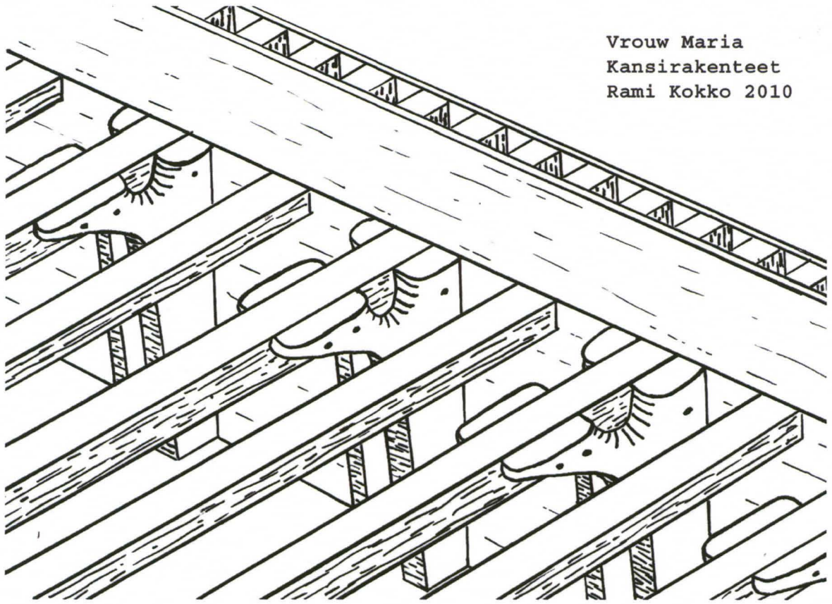
Kuva 5.2.1. Perspektiivipiirros Vrouw Maria -hylvn kansirakenteista paapuuriinpuoleisella laidalla. Kansilankut on jätetty pois piirrokselta runkorakenteiden havainnoinnin helpottamiseksi. Piirros Rami Kokko, Museovirasto.
