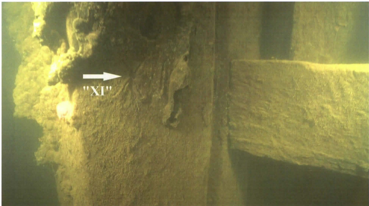
Kuva 5.2.2. Perärangan pinnassa erottuva merkintä "XI". Kaappauskuva Juha Flinkmanin kuvaamasta videosta MA201014:57. Kuvankäsittely Rami Kokko.
