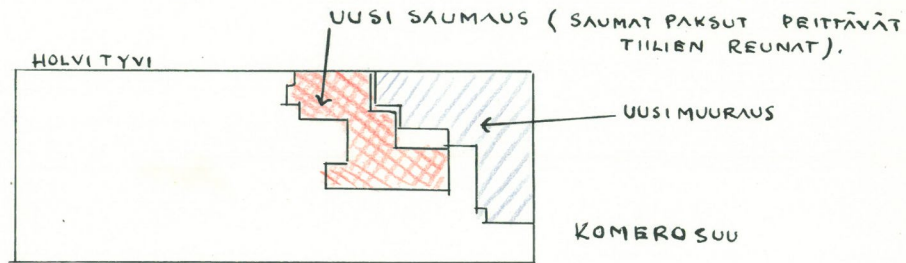
LÄNSISEINÄ
