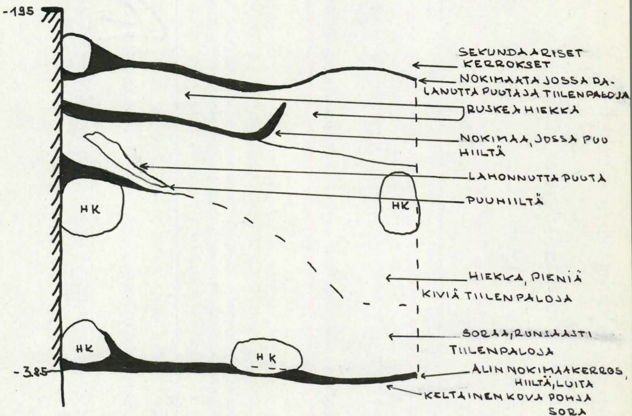
LEIKKAUS SAMASTA
