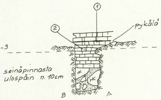
Leikkaus A-B
