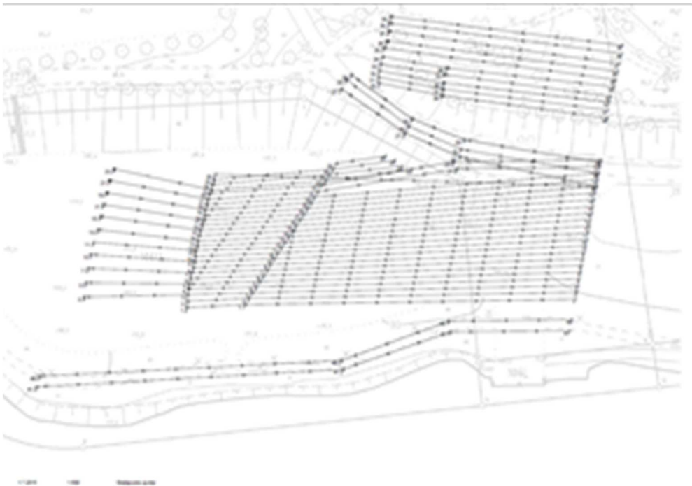
Kuva 15. Frenckellin kalkkiruukin alueelle mitatut maatutkaluotauslinjat.
