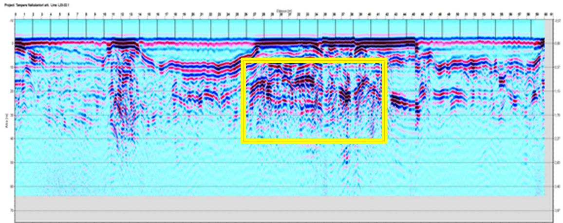
Kuva 16. Kuva Nalkalantorin maatutkaluotausprofiilista nro 33, johon mahdollisesti arkeologisesti mielenkiintoinen ilmiö on merkitty keltaisen laatikon sisään. (Kuva: Pollari 2015; merkintä Kirsi Luoto Risto Pollarin mukaan)
