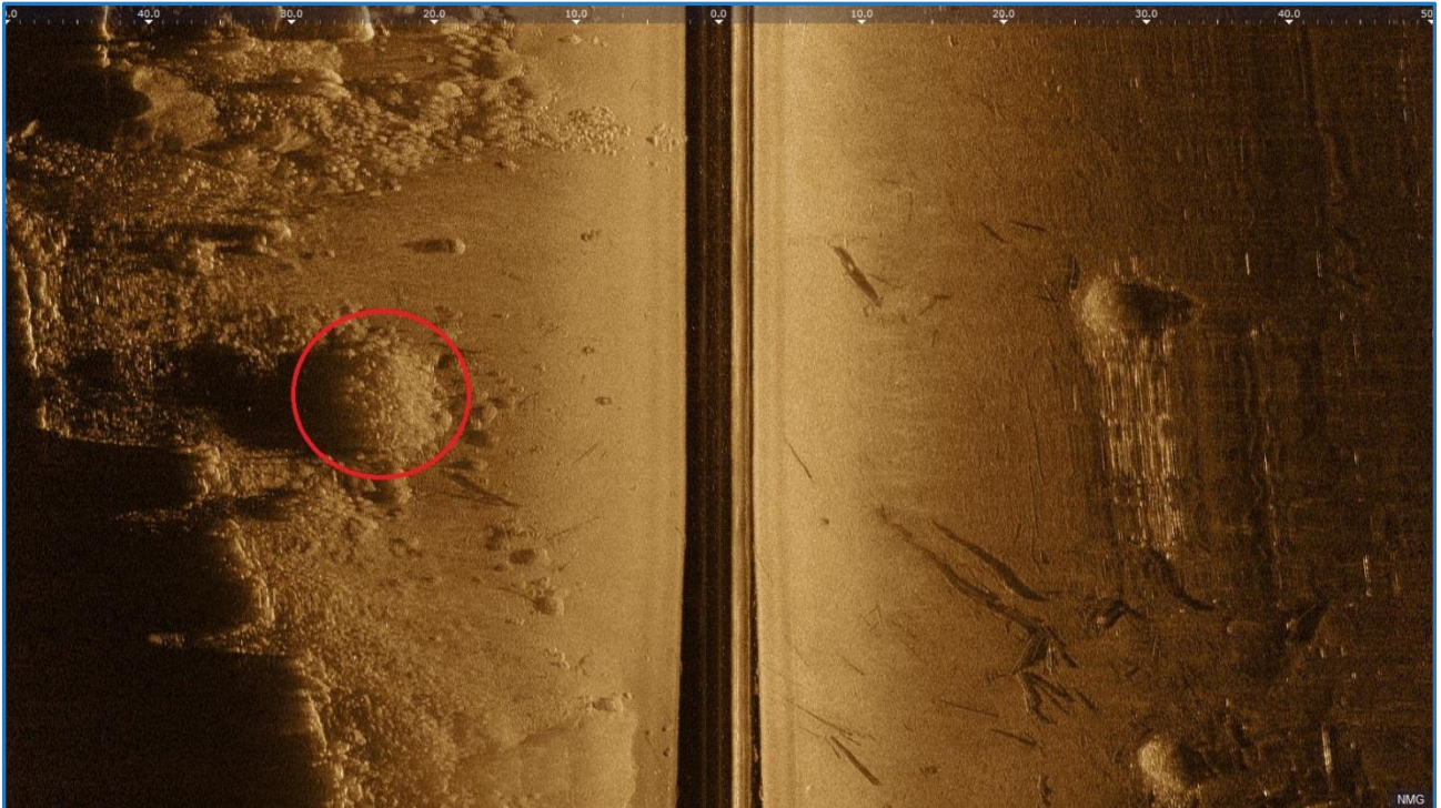
Kuva 34. Viistokaikuluotauskuva kohteesta 7.
