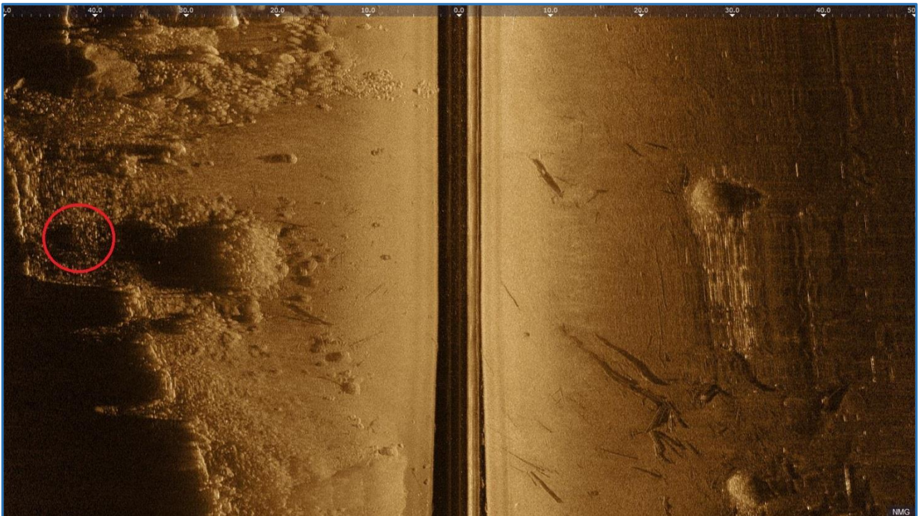
Kuva 32. Viistokaikuluotauskuvat kohteesta 6.
